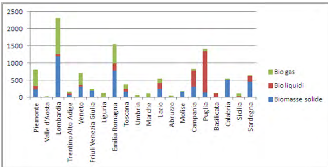
F21 - Fig.1– Produzione di energia elettrica (GWh) da bioenergia nelle Regioni Italiane- anno 2011 (ICS 67)
